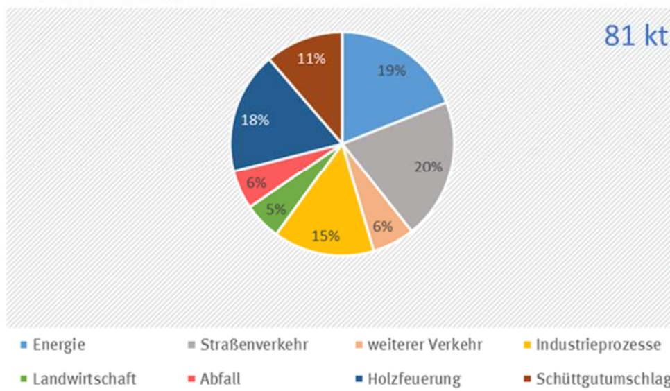
Zusammensetzung der nationalen PM 2,5 -Emissionen 2020 nach Berichterstattung 2022
